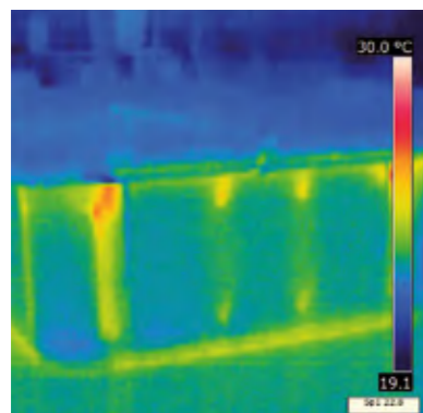
Warmtelekttest uitgevoerd met het Nordic Insulation System
